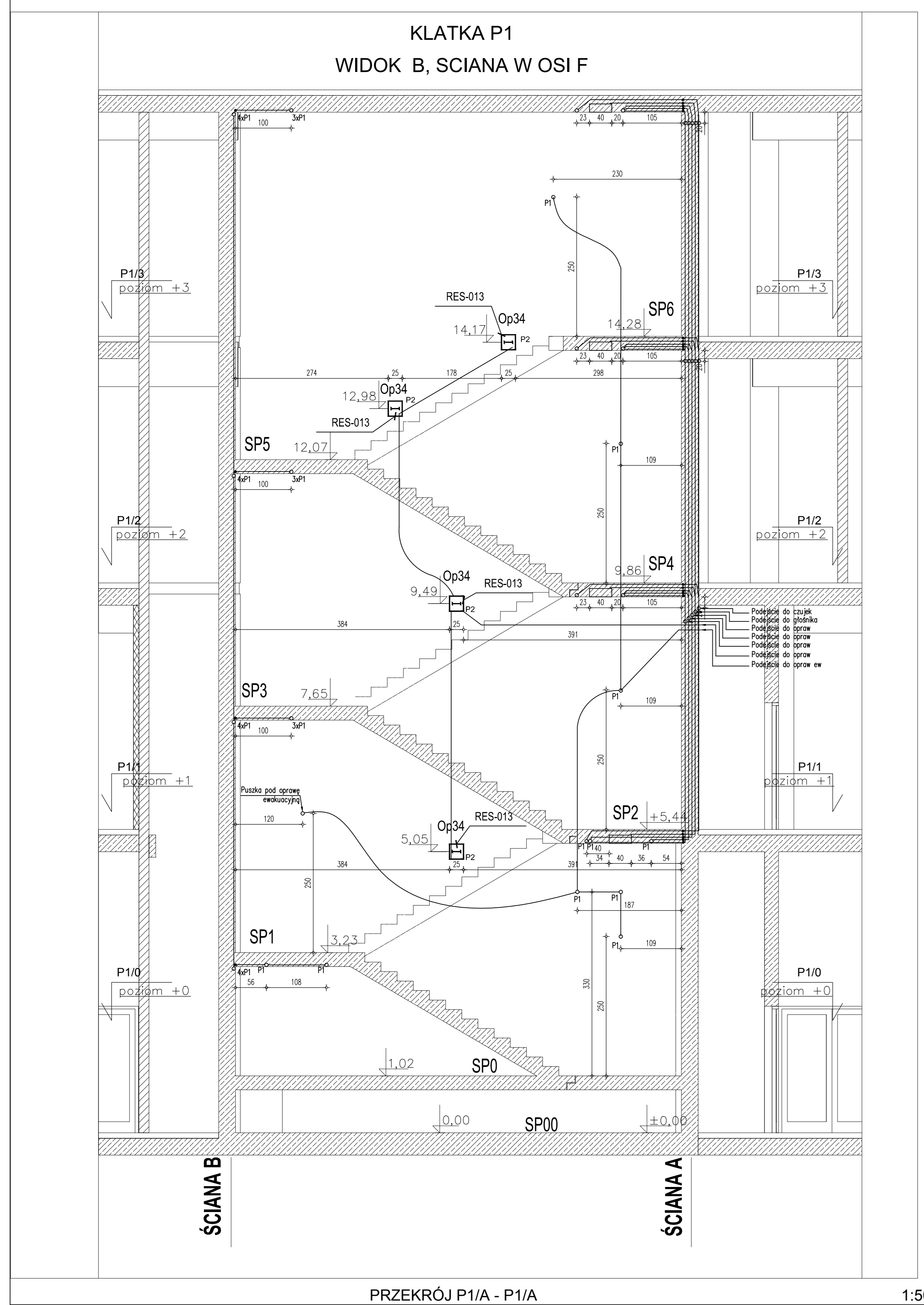
PRZEKRÓJ P1/A - P1/A 1:50
