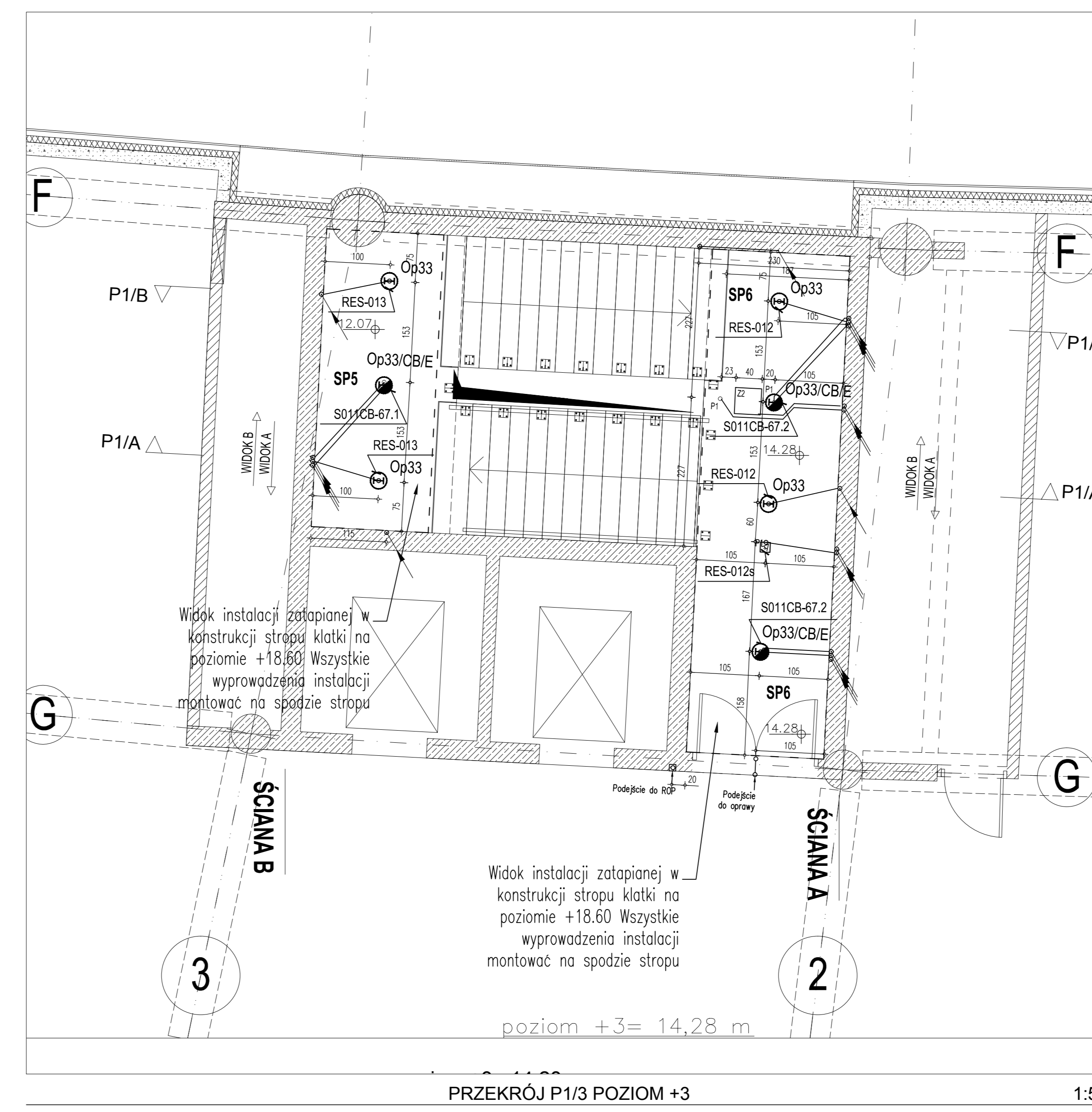
PRZEKRÓJ P1/3 POZIOM +3 1:50
