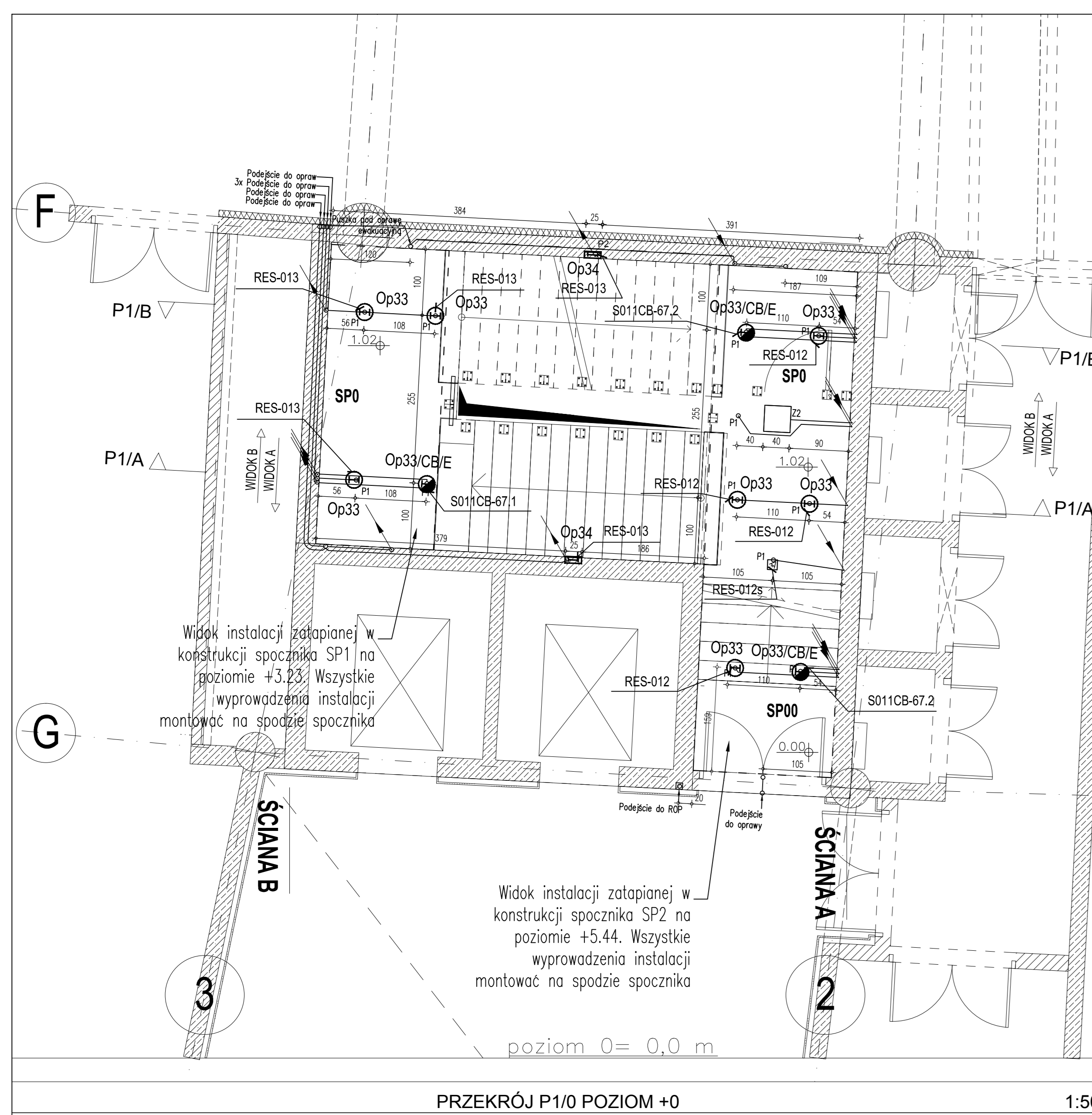
PRZEKRÓJ P1/0 POZIOM +0 1:50
