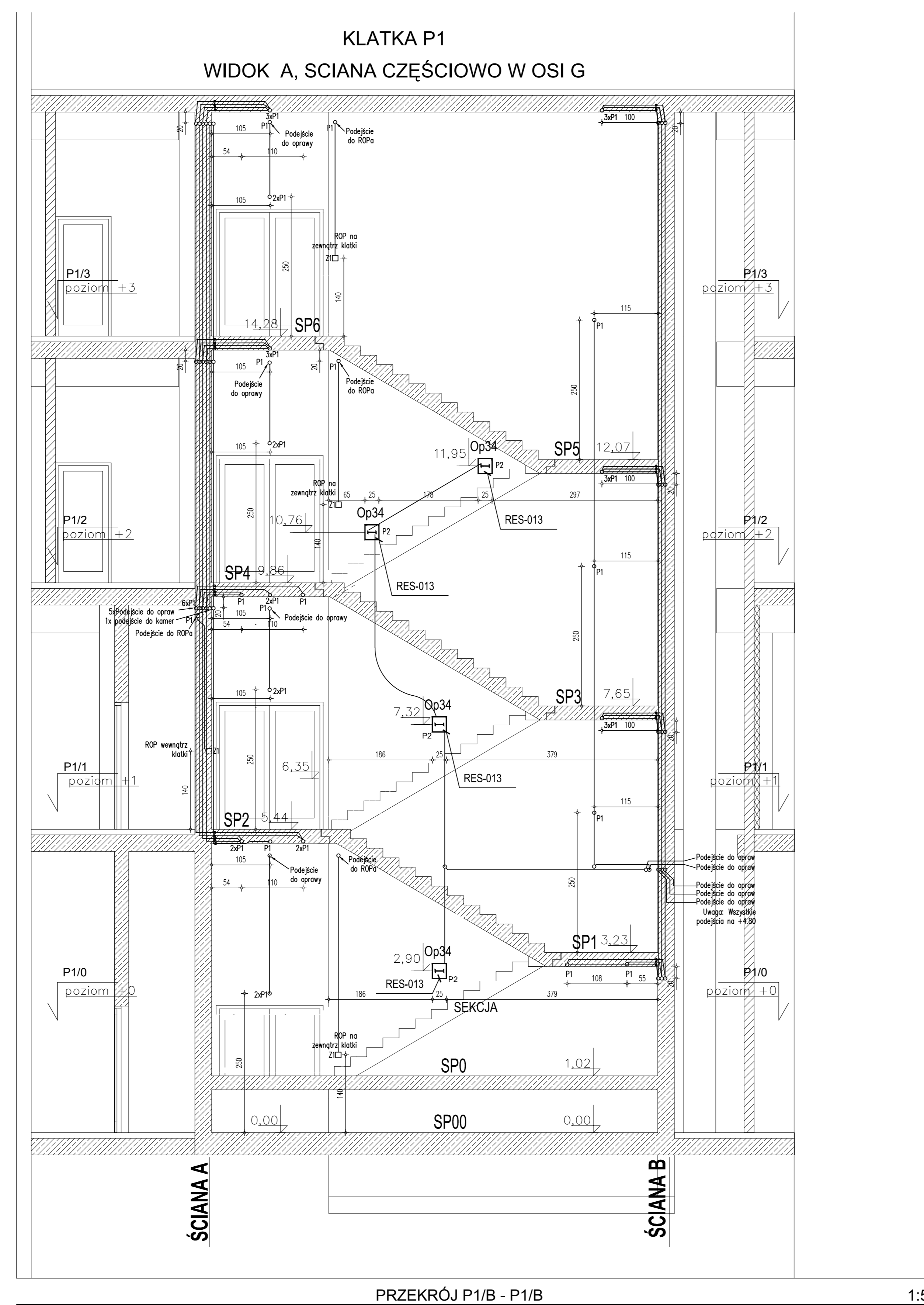
PRZEKRÓJ P1/B - P1/B 1:50
