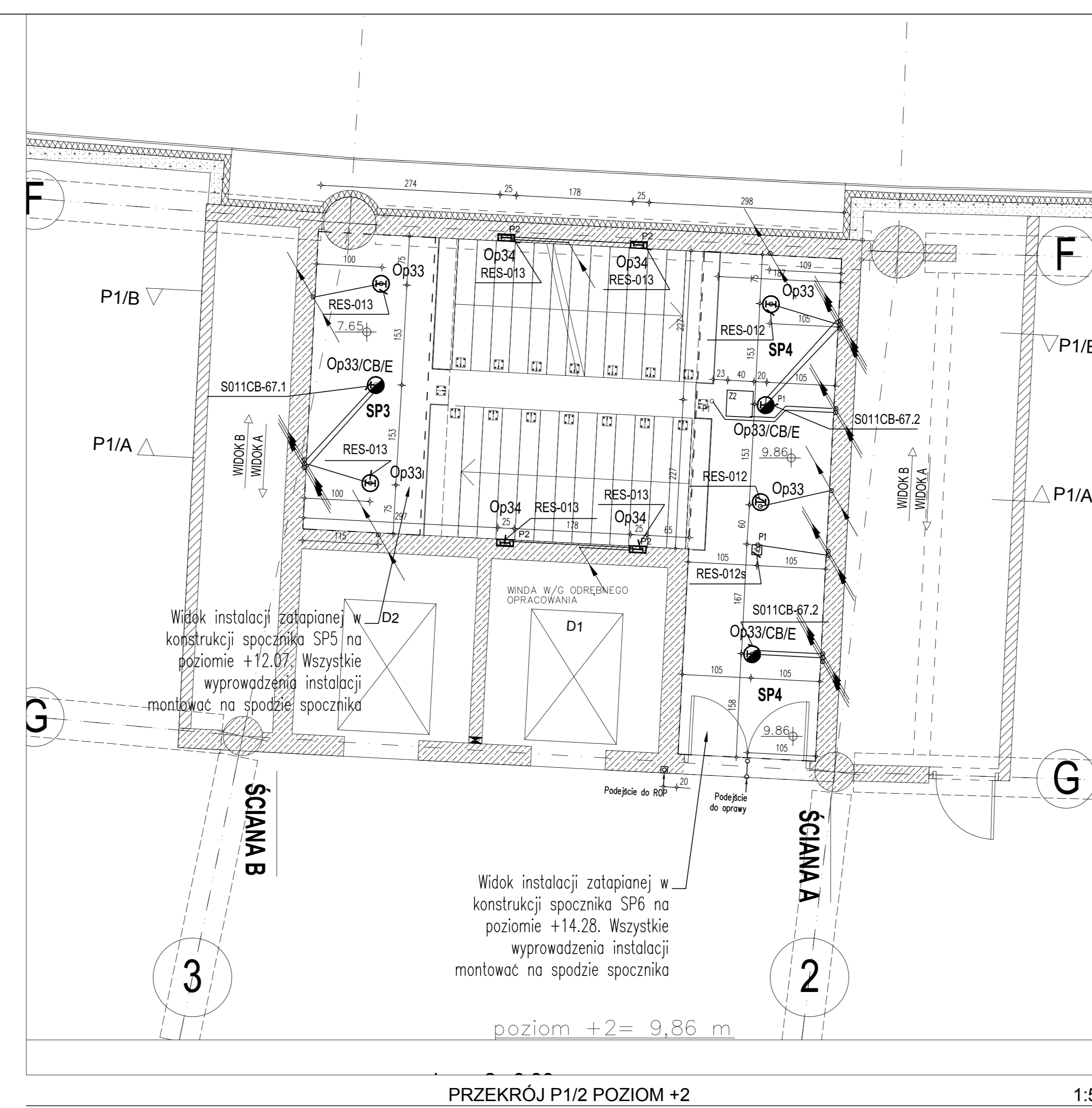
PRZEKRÓJ P1/2 POZIOM +2 1:50
