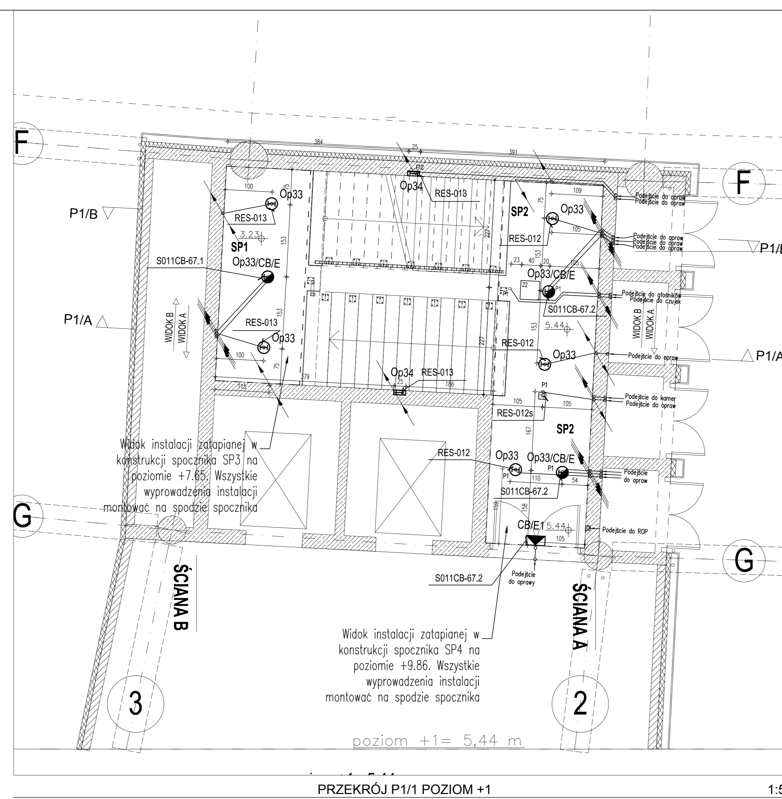
PRZEKRÓJ P1/1 POZIOM +1 1:50
