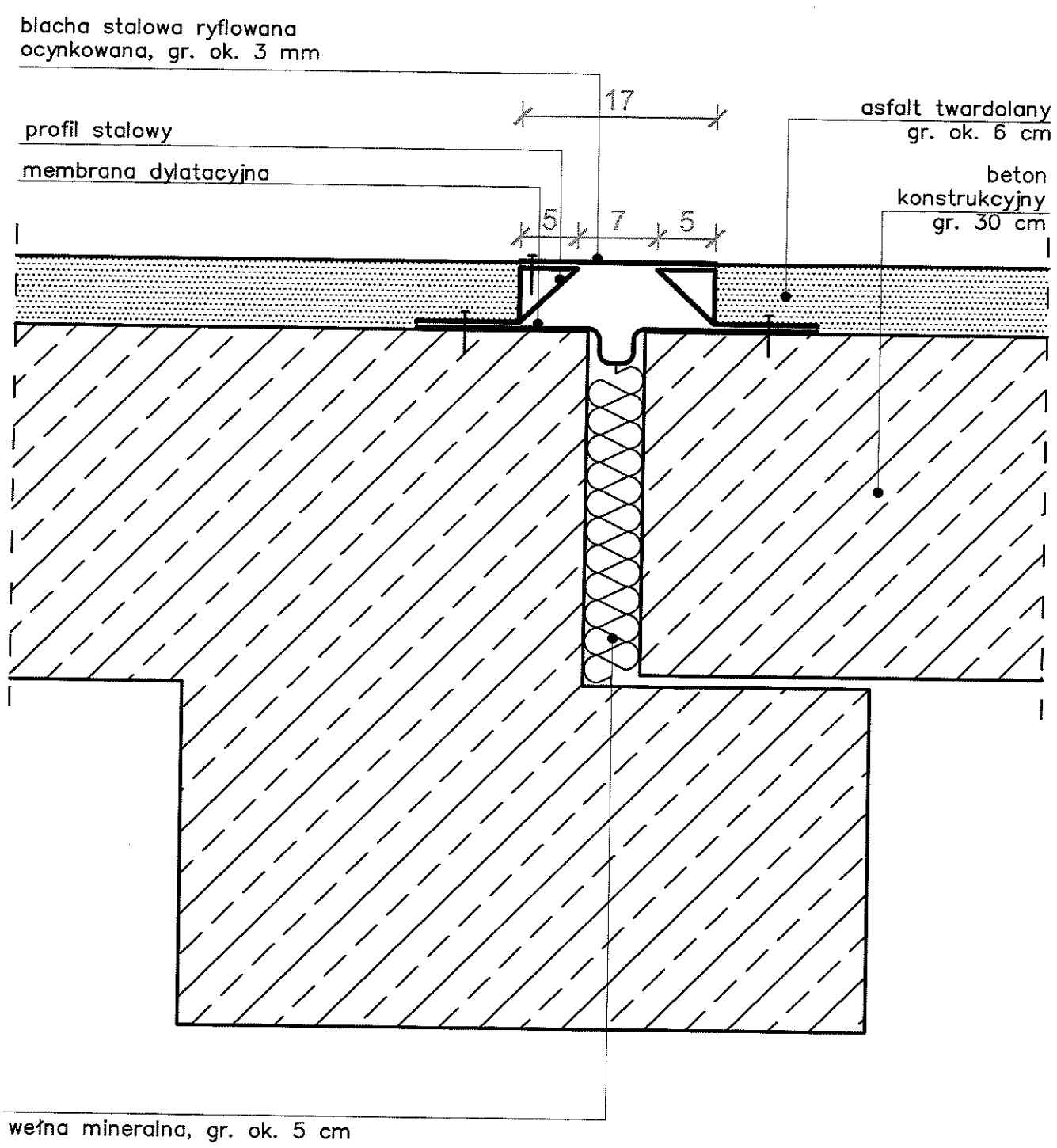
Rys. 2 Przekrój przez szczelinę dylatacyjną- typ II
